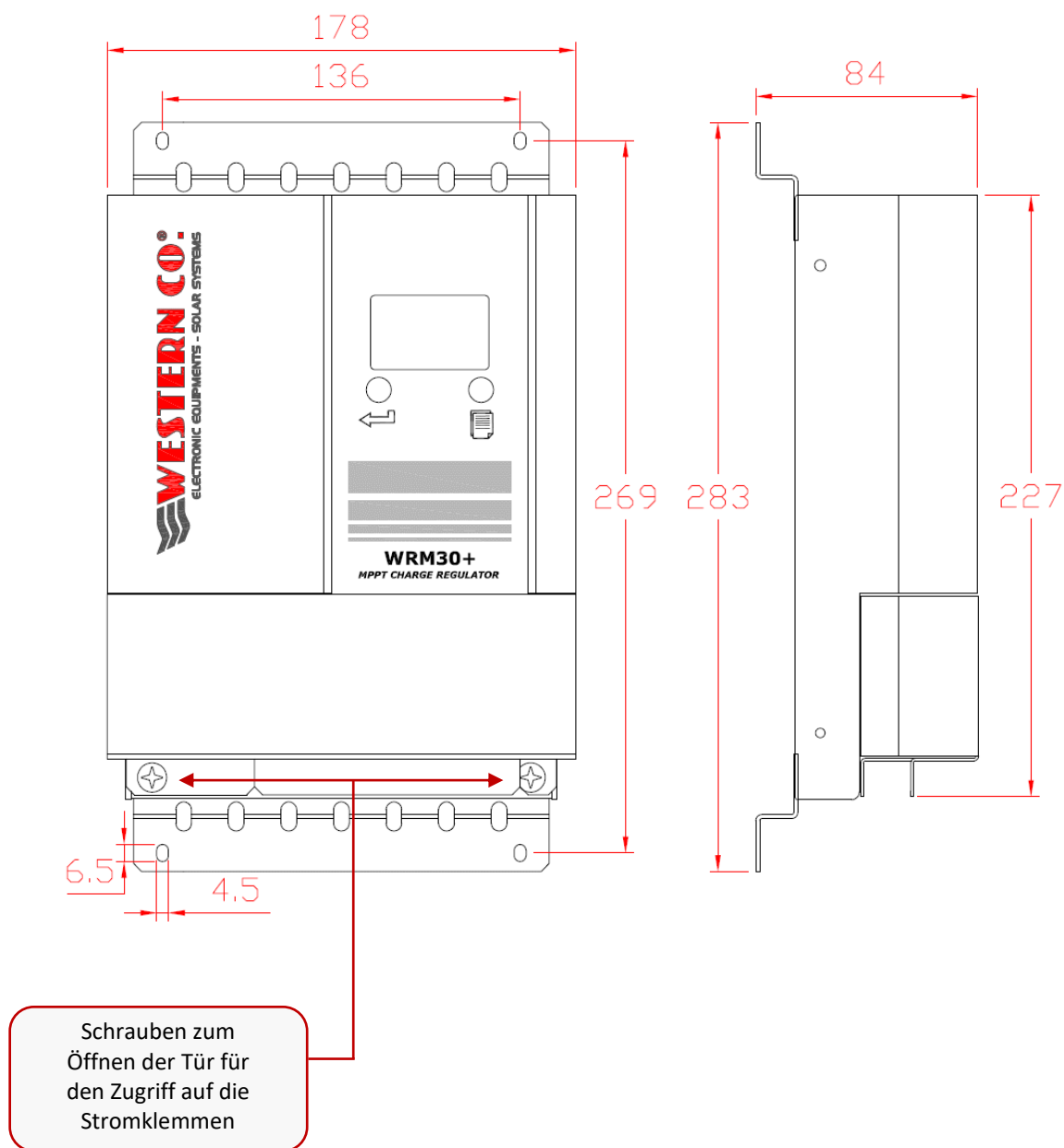
Abb. 4 Ausmaße (mm)
