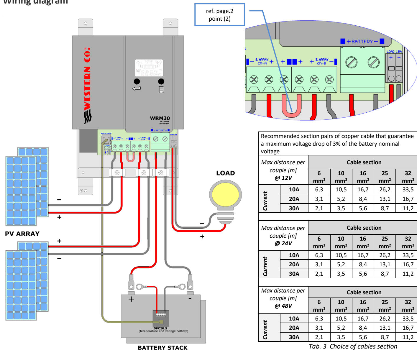
Fig. 2 Wiring diagram
