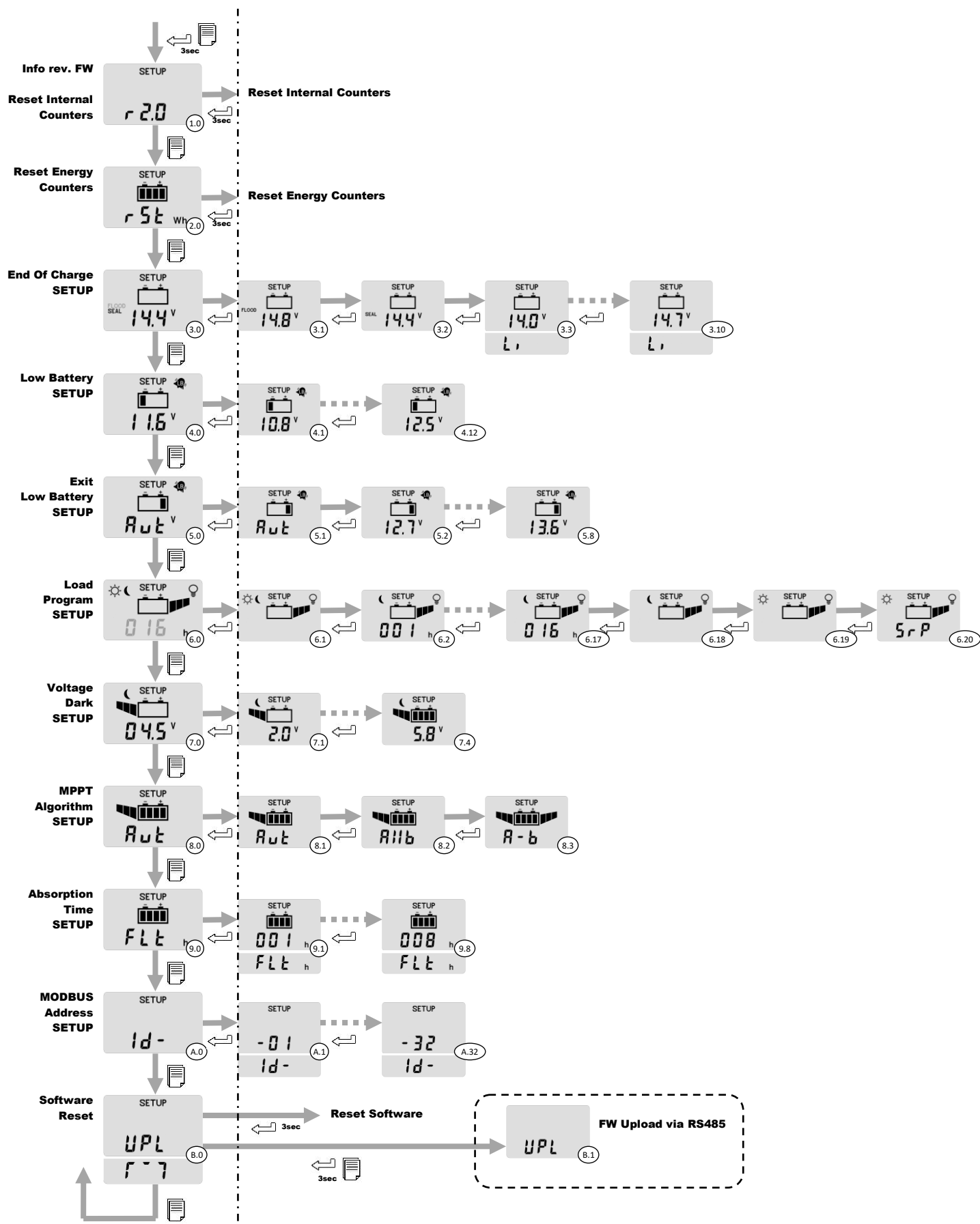
Fig. 6 Schéma de navigation dans le menu SETUP
