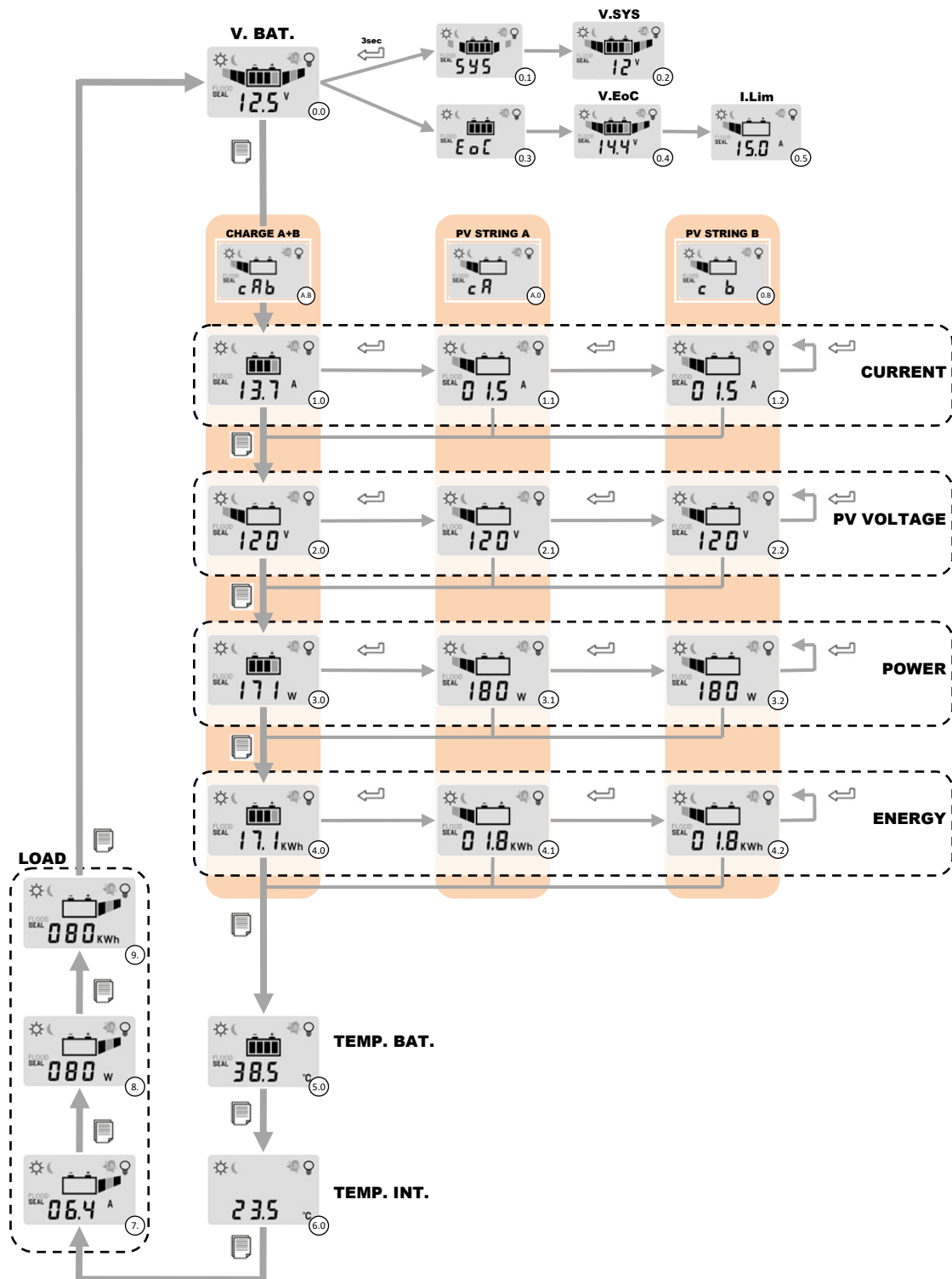
Abb.5 Navigationsschema menü
