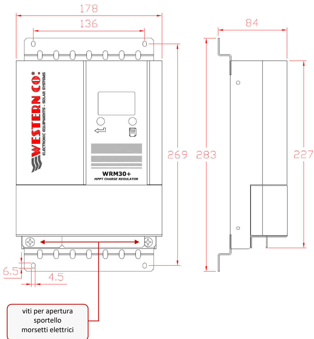
Fig. 4 Dimensioni (mm)
