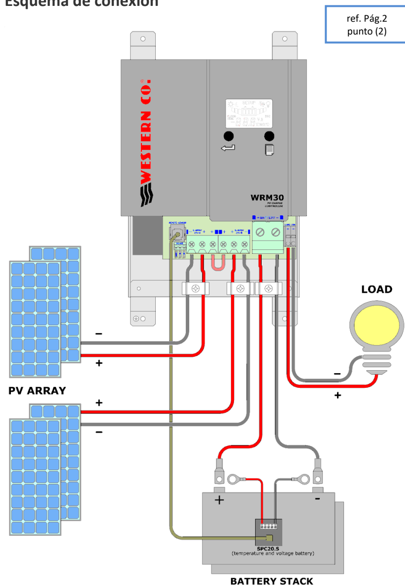
Fig. 2 Esquema de conexión
