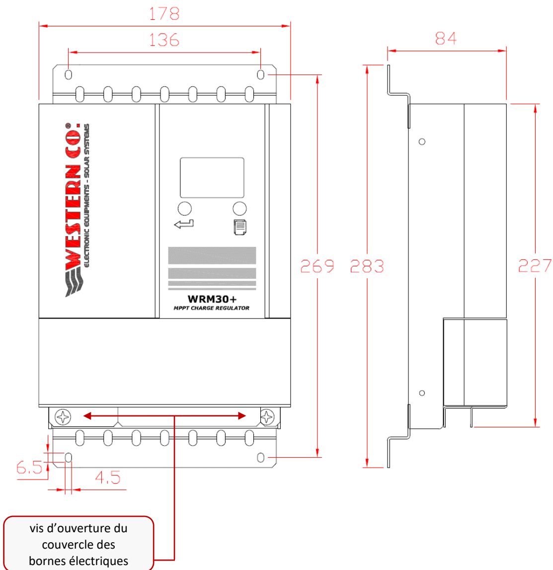
Fig. 4 Dimensions (mm)
