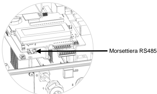
Figura 21: Morsettiere RS485
