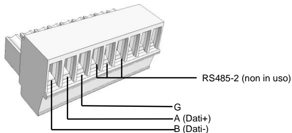
Figura 22: Morsetteria RS485
