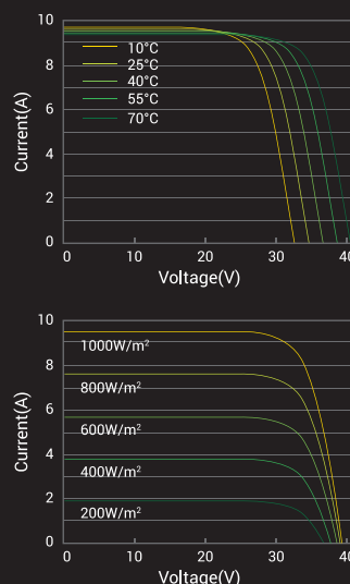
I-V Curve: (A-M400)
