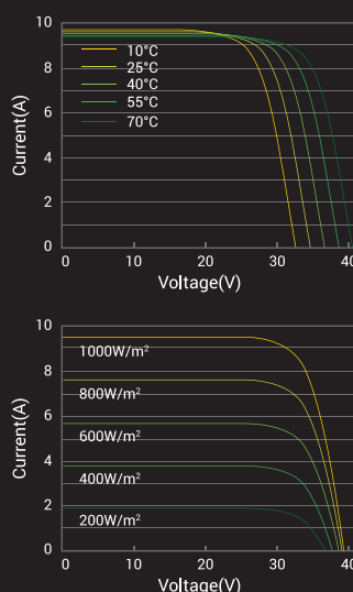
I-V Curve: (A-HCM350)
