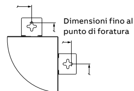
Veduta frontale Fissaggio esterno Dettaglio
