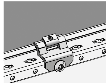
Continuità elettrica delle parti mobili garantita dalla speciale conformazione delle cerniere
